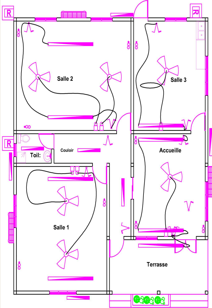
PLAN D'ELECTRICITE
